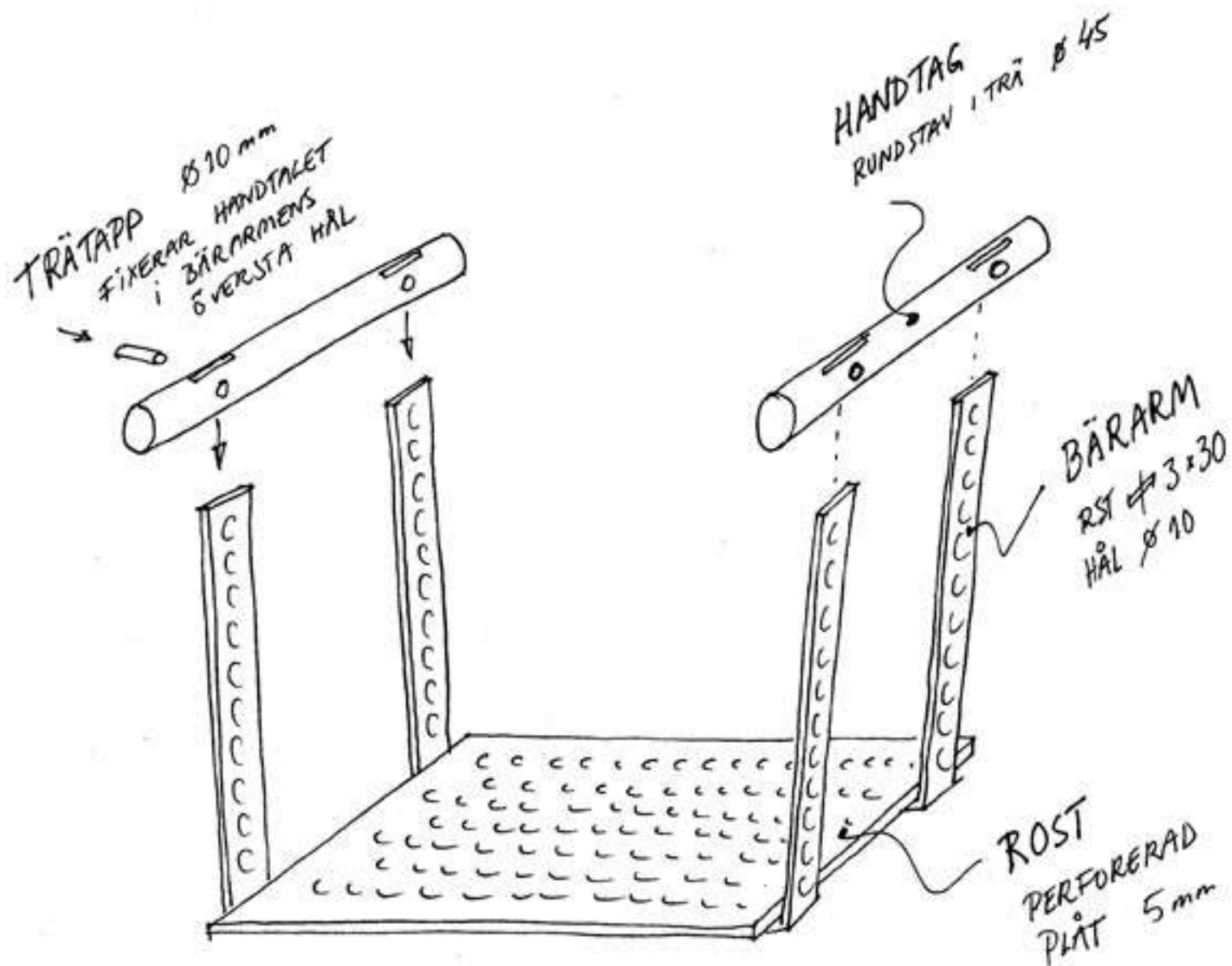
PRINCIPSSKISS ÖVER ROST MED BÄRARMAR OCH HANDTAG
